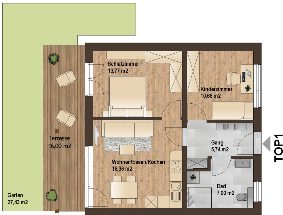
Grundriss
